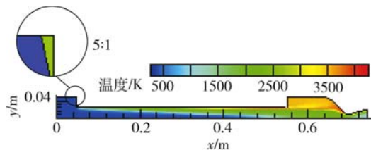
图 4 发动机内部温度云图(前燃室 0.75d_c )
