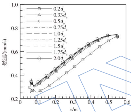
图 5 不同长度前燃室燃速沿轴向分布
