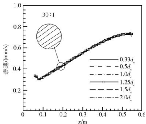
图 7 不同长度后燃室燃速沿轴向分布
