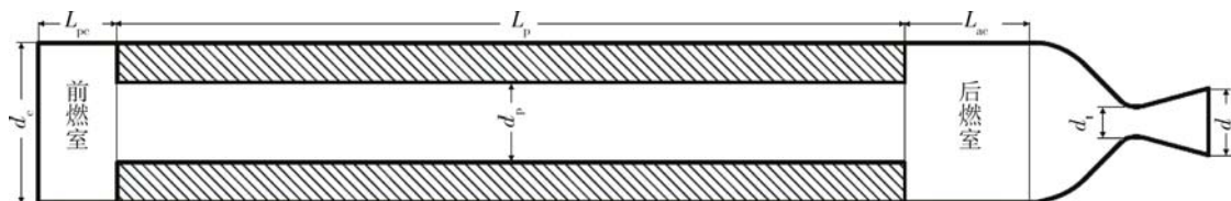
图 2 发动机结构图
