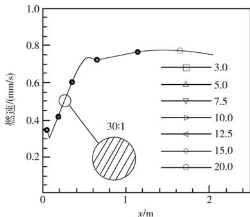
图9 不同长径比药柱的燃速沿轴向分布
