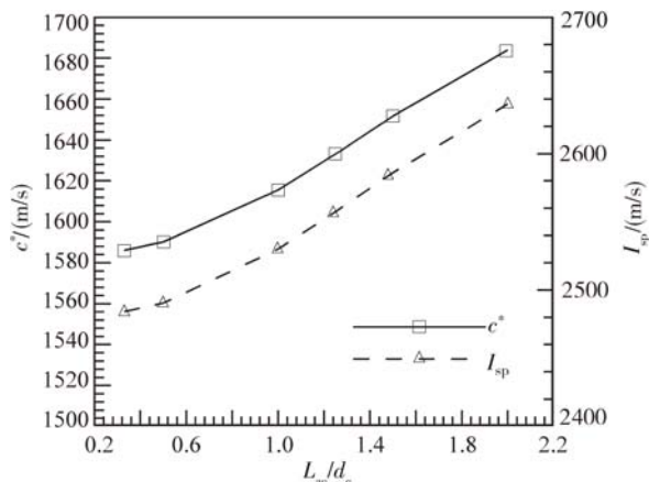
图8 不同长度后燃室的特征速度与真空比冲变化曲线
