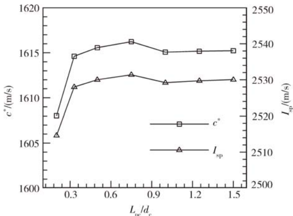
图 6 不同长度前燃室的特征速度与真空比冲变化曲线
