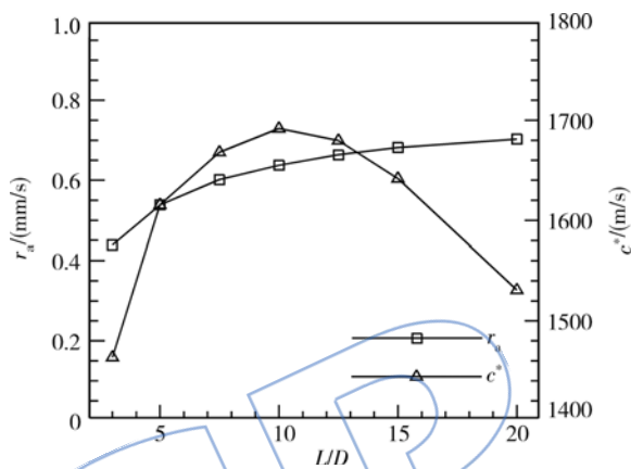
图10 不同长径比药柱的平均燃速与特征速度变化曲线
