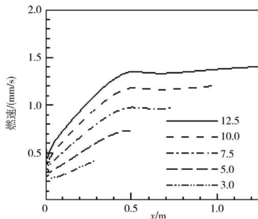
图 11 不同长径比药柱的燃速沿轴向分布
