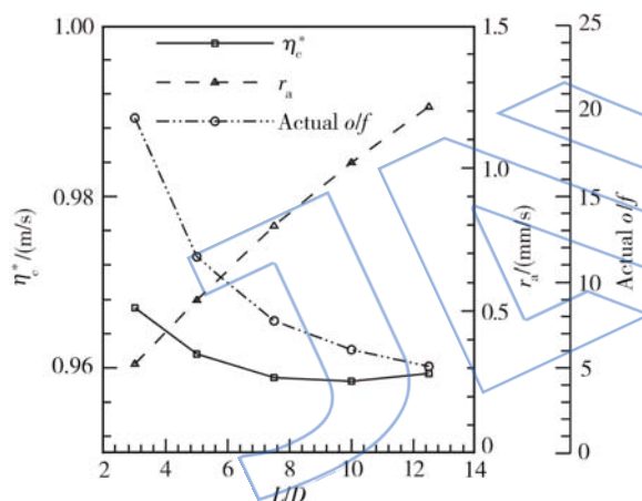
图 12 燃烧效率、平均燃速和实际氧燃比随药柱长径比变化曲线
